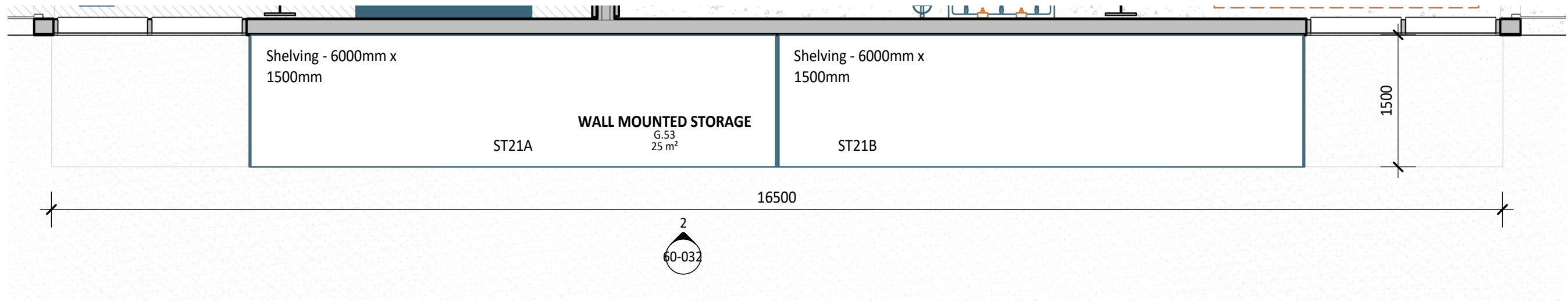
1 PLAN DETAIL 1 : 50
